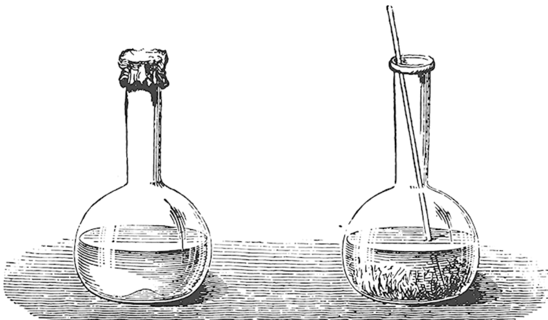
Осаждение
