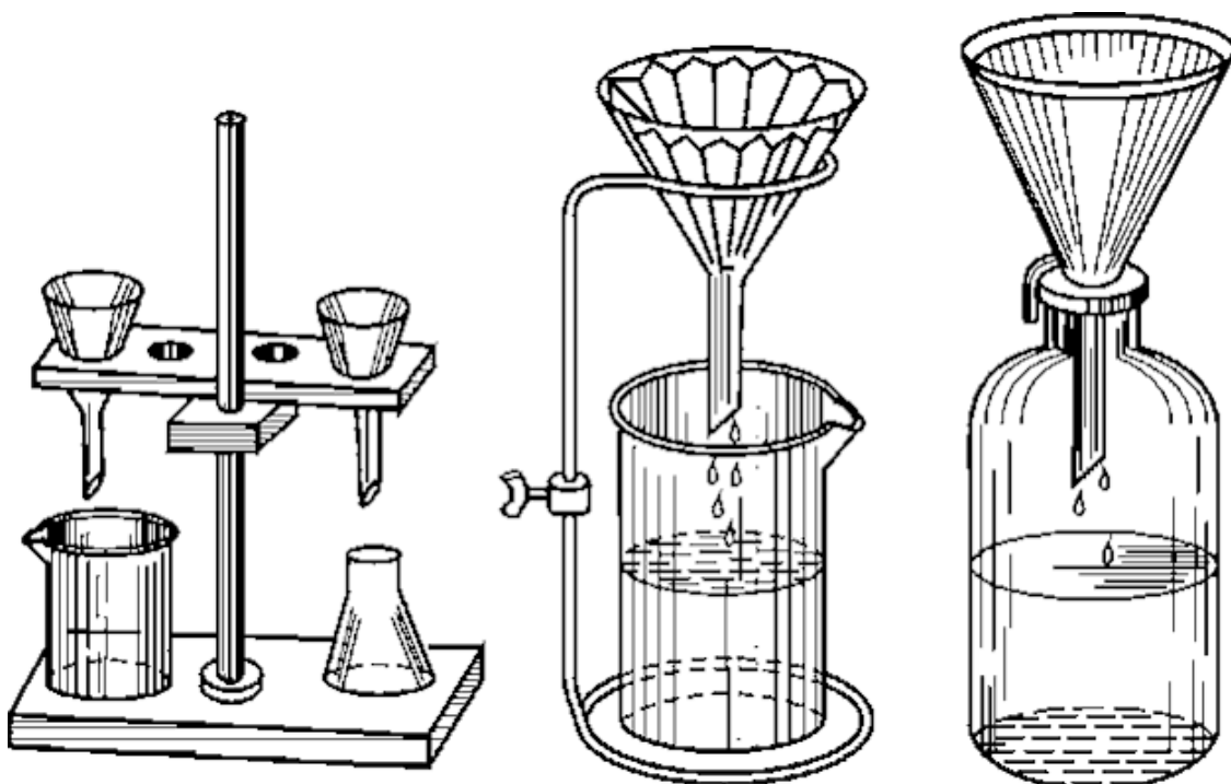
Фильтрация
