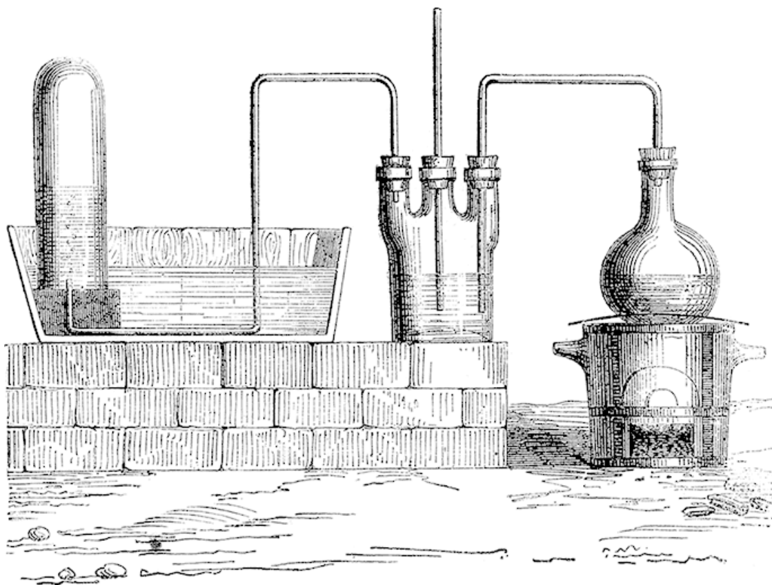
Возгонка
