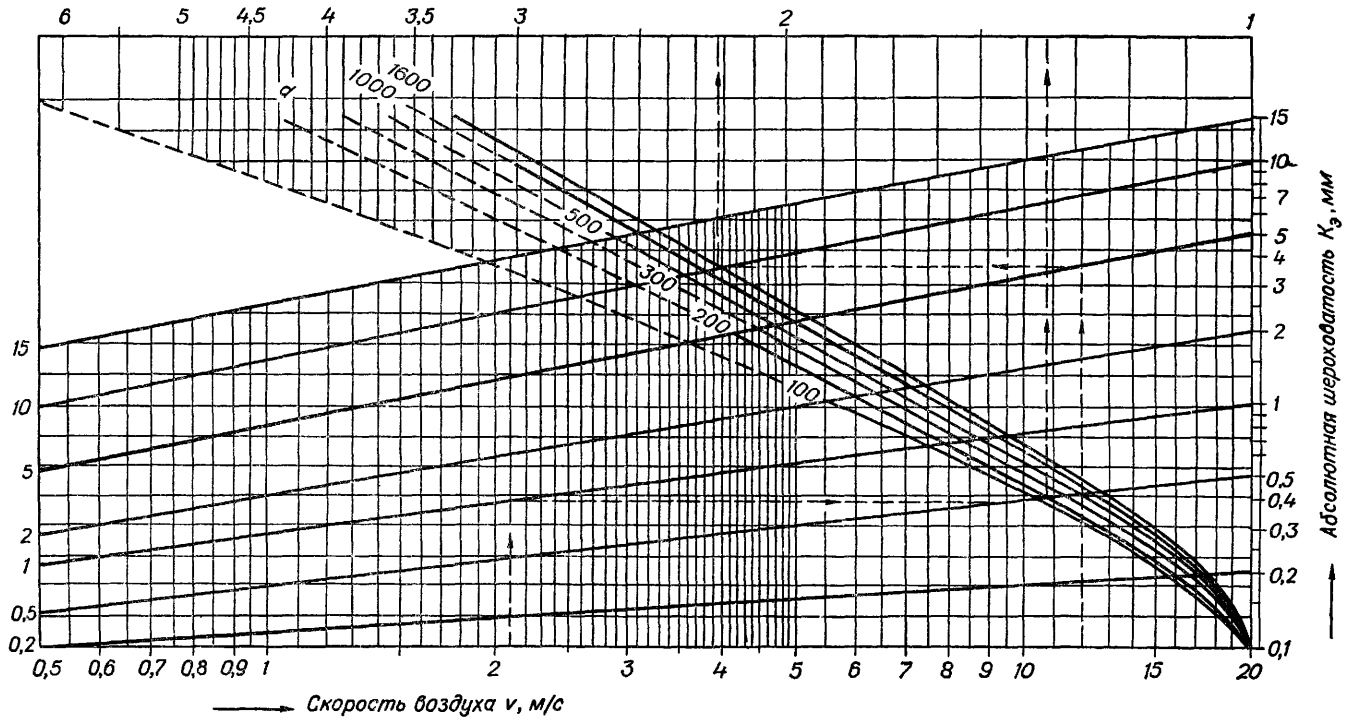
Лист VII.12. Номограмма для определения поправочного коэффициента n шероховатых воздуховодов.
