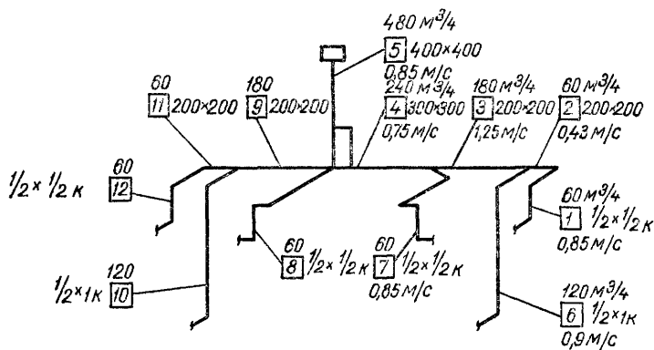
Лист VII.1. Схема вентиляции зрительных залов (рис. 1) и расчетная схема к примеру VII.2 (рис. 2):
