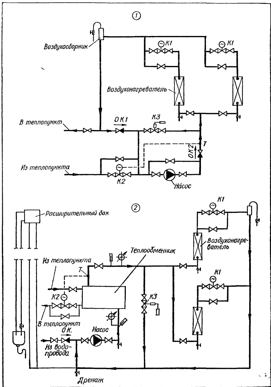
Лист VIII.18. Принципиальные схемы теплоснабжения calorиферов второго, местного и зонального подогрева:
