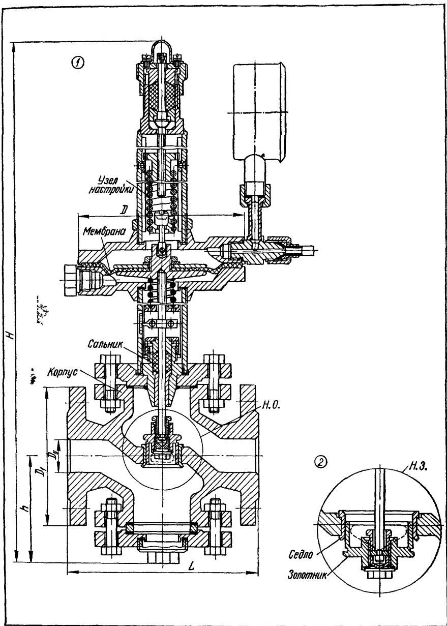
Лист IX.1. Клапан типа ПК-1: 1 — клапан сборки Н.О.; 2 — узел золотника сборки Н.З.
