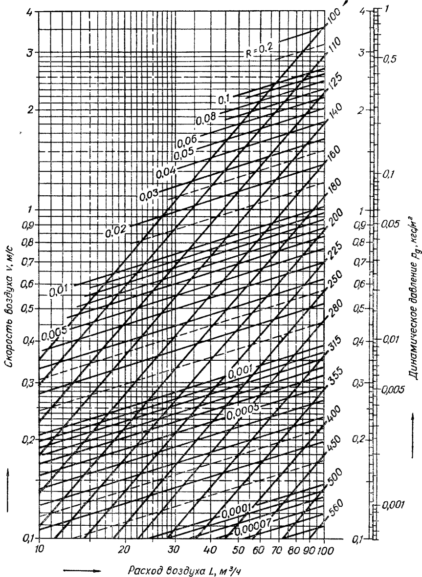
Лист VII.7. Номограмма для расчета круглых стальных воздухопроводов при расходах воздуха до 100 м 3 /ч (при K = 0,1 ; \gamma = 1,2 кг/м 3 ).
