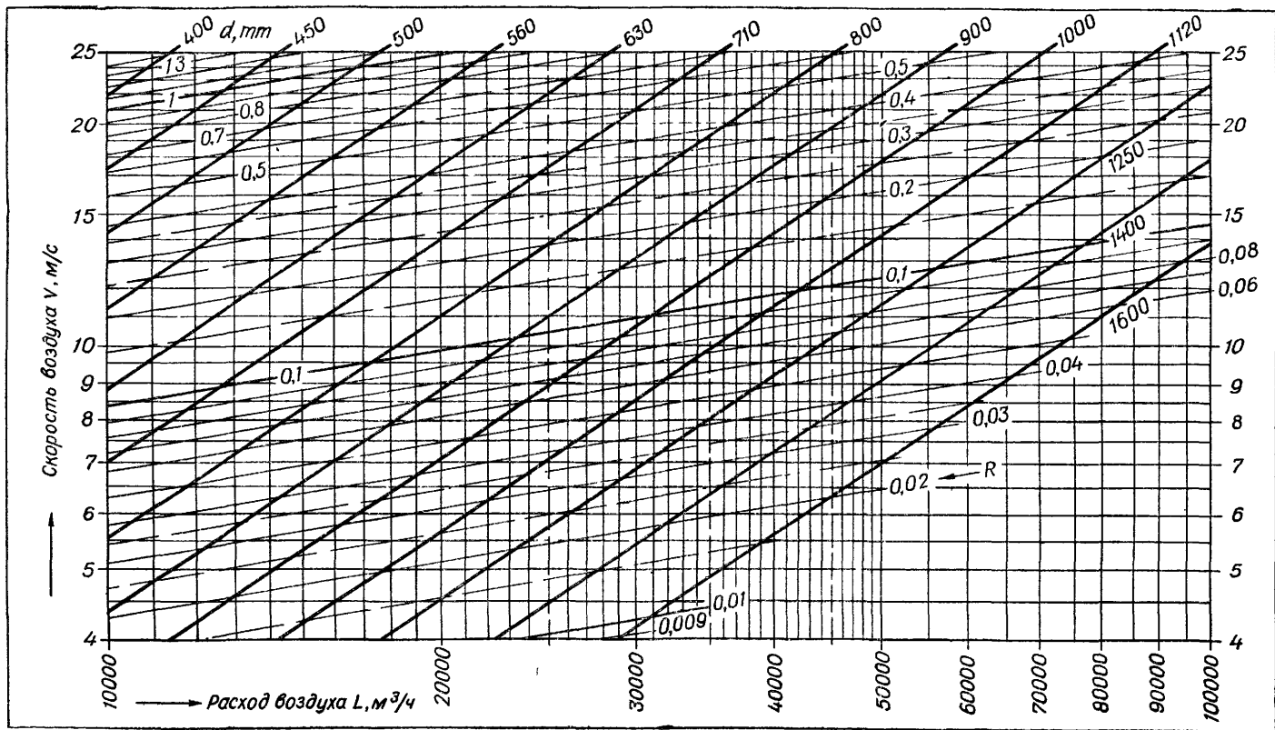
Лист VII.10. Номограмма для расчета круглых стальных воздухопроводов при расходах воздуха от 10 000 до 100 000 \text{м}^3/\text{ч} и скорости воздуха от 4 до 25 \text{м/с} (при K = 0,1 , \gamma = 1,2 \text{ кг/м}^3 ).
