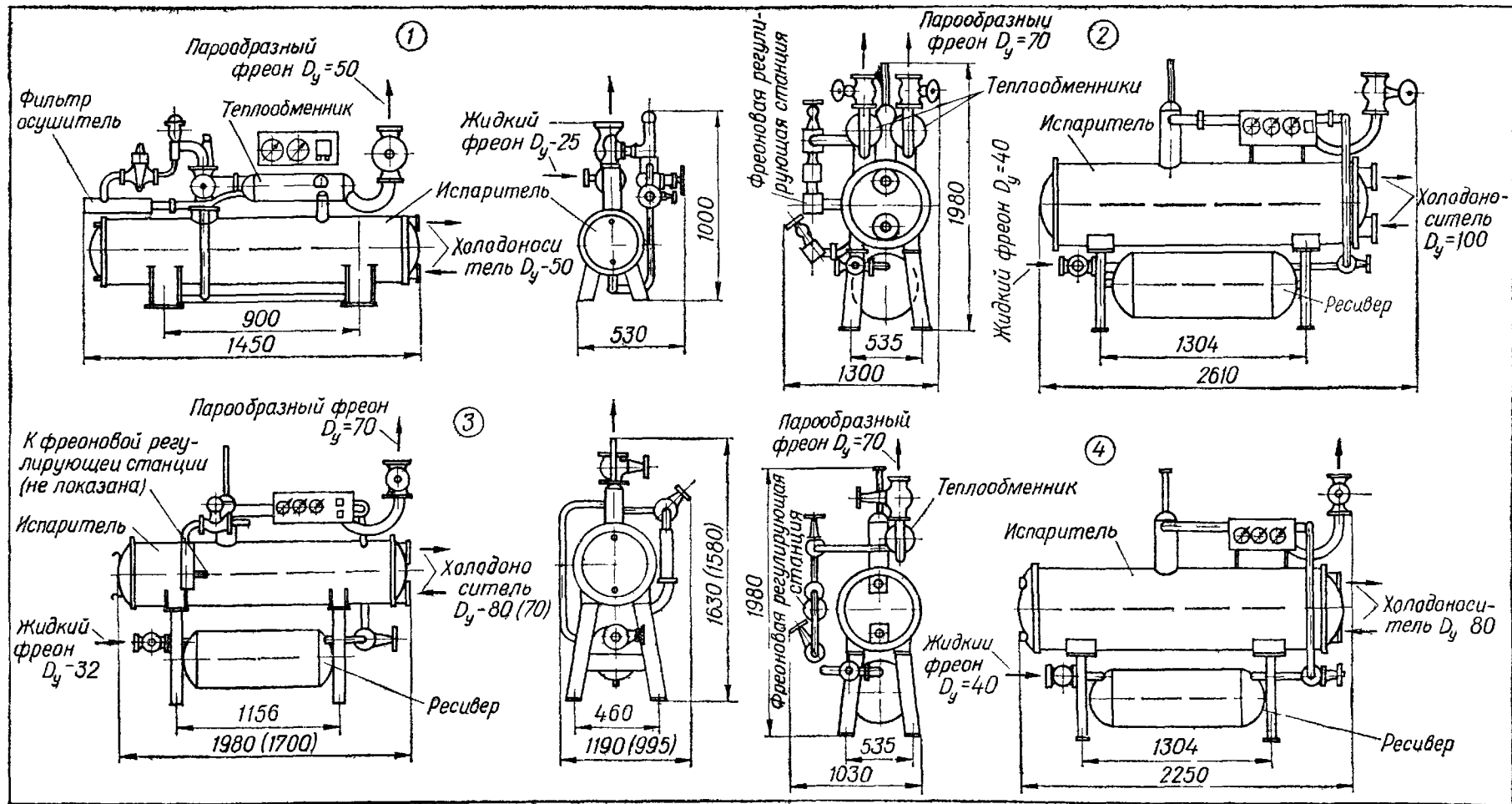
Лист VIII.22. Испарительно-регулирующие агрегаты:
