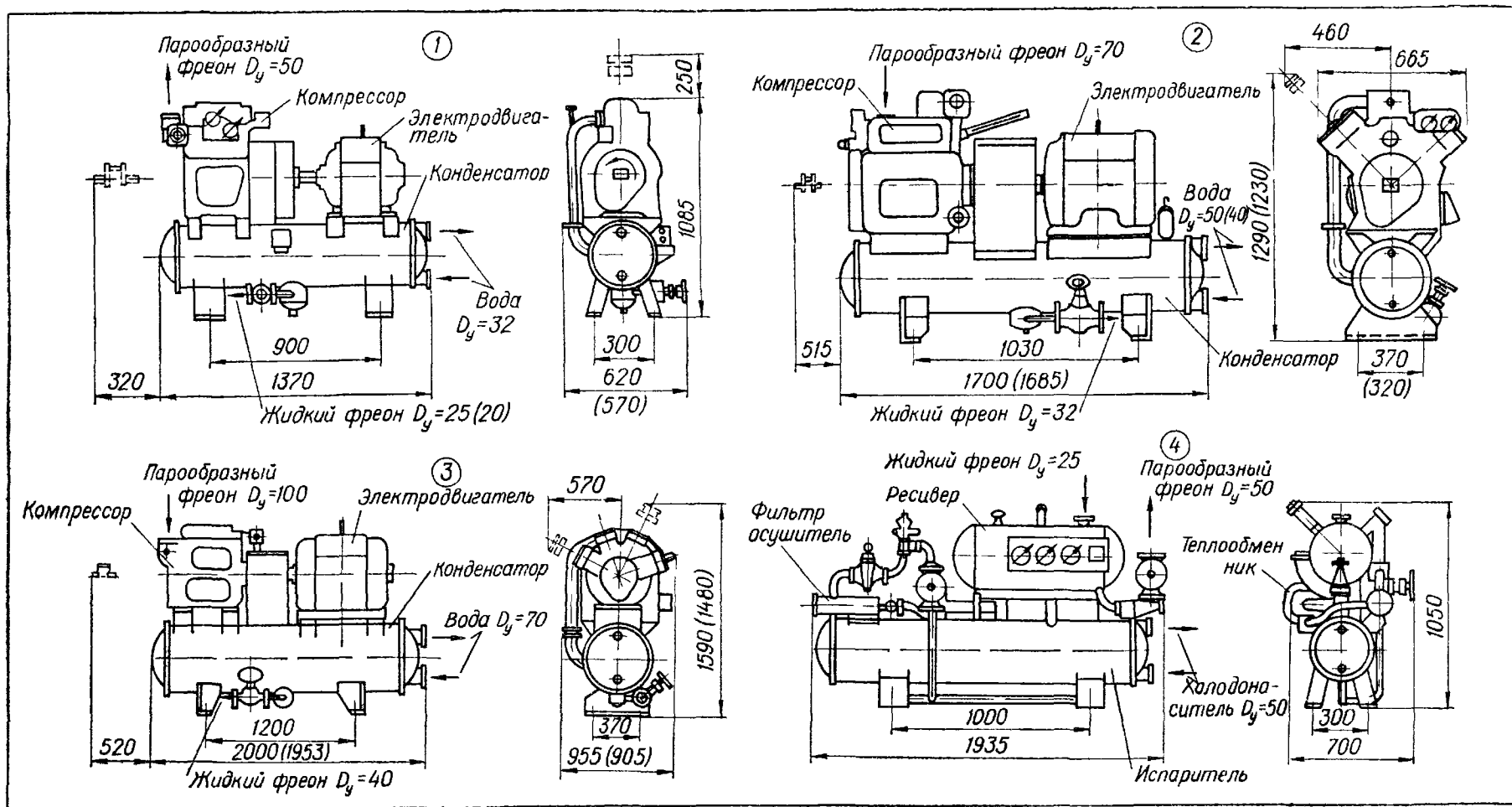
Лист VIII.21. Агрегаты холодильных машин:
