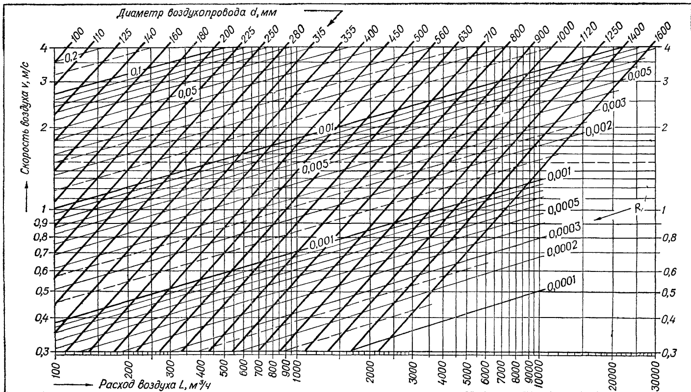
Лист VII.8. Номограмма для расчета круглых стальных воздухопроводов при расходах воздуха от 100 до 10 000 м 3 /ч и скорости воздуха от 0,3 до 4 м/с (при K = 0,1 , \gamma = 1,2 кг/м 3 ).
