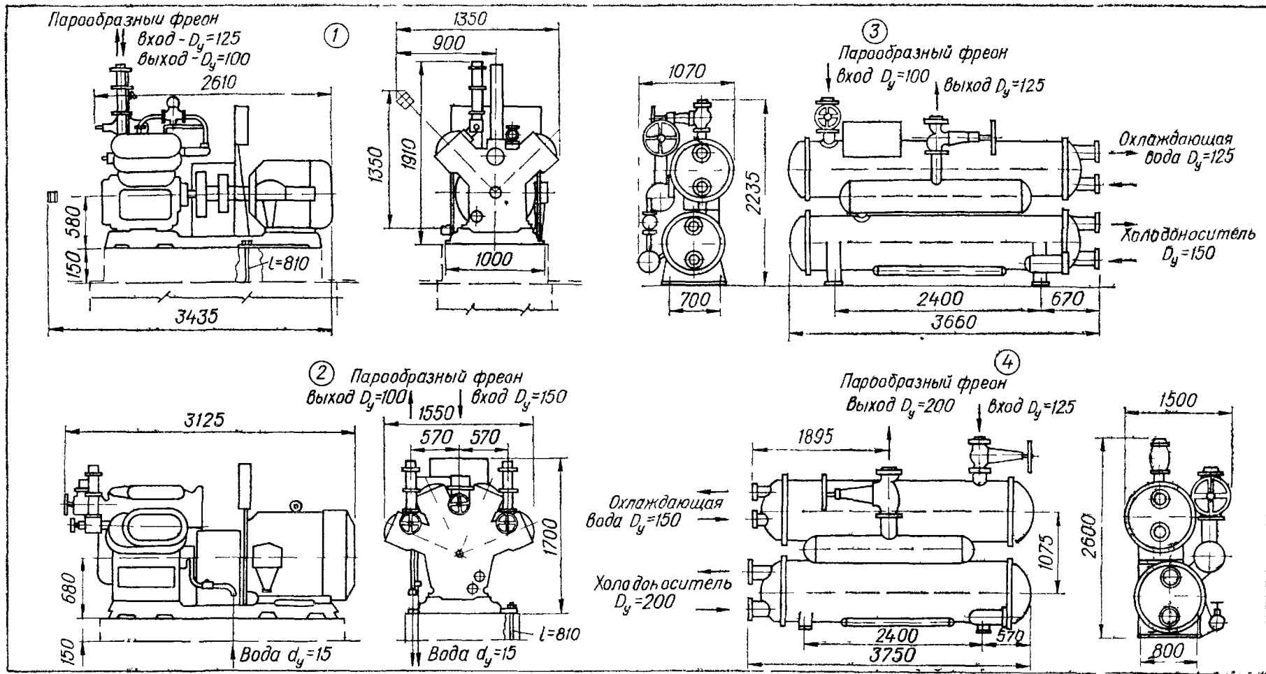
Лист VIII.23. Агрегаты холодильных машин:
