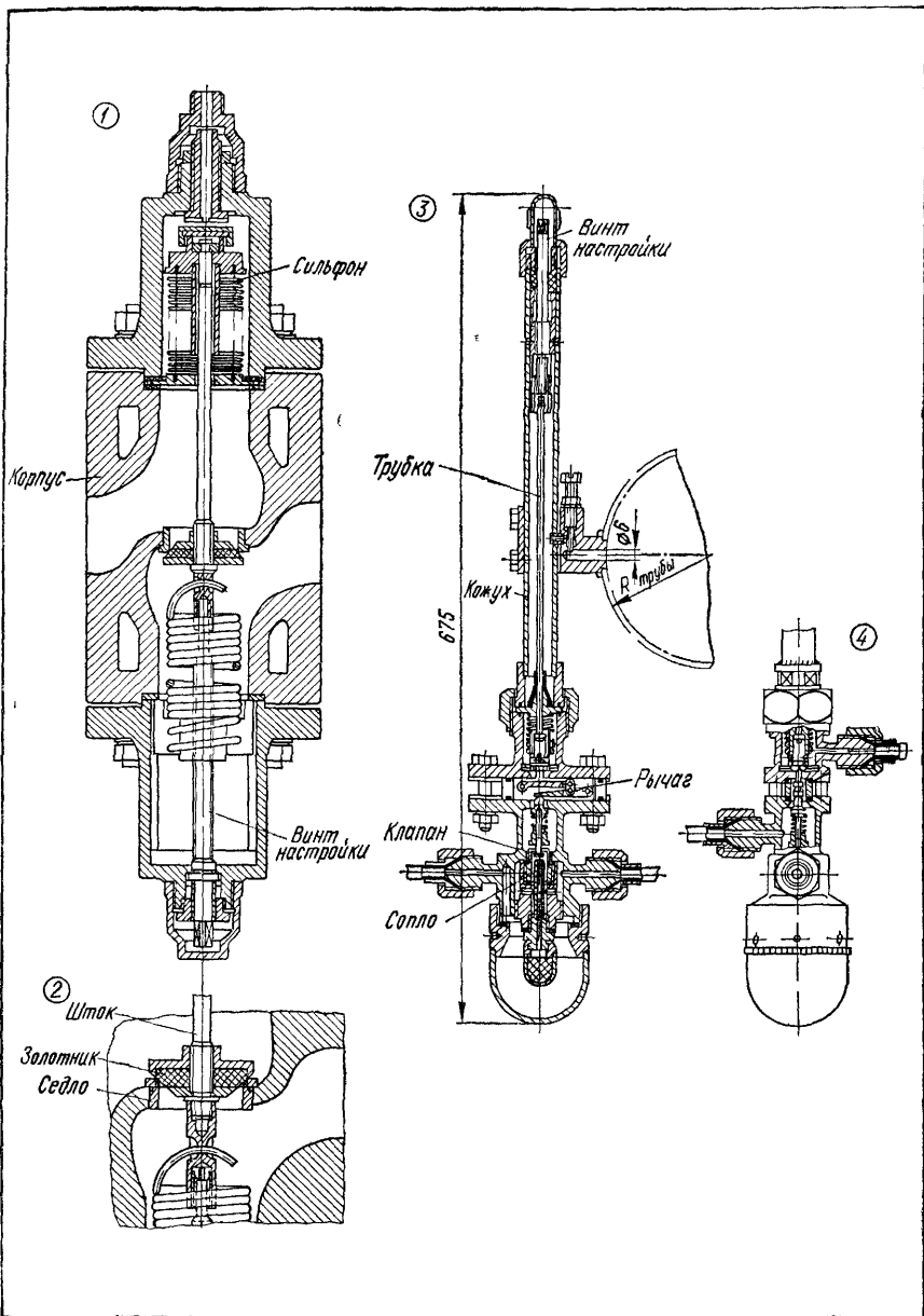
Лист IX.3. Гидравлические регуляторы расхода давления и температуры: 1 — регулятор расхода типа РР; 2 — сборка золотника регулятора давления типа РД; 3 и 4 — регулирующий прибор типа ТРД.
