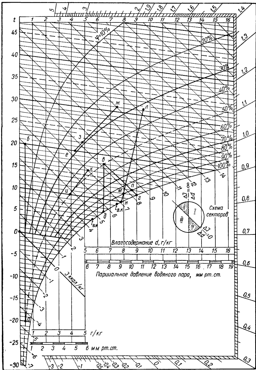
Лист VII.14. Построение процессов обработки воздуха в I - d -диаграмме:
