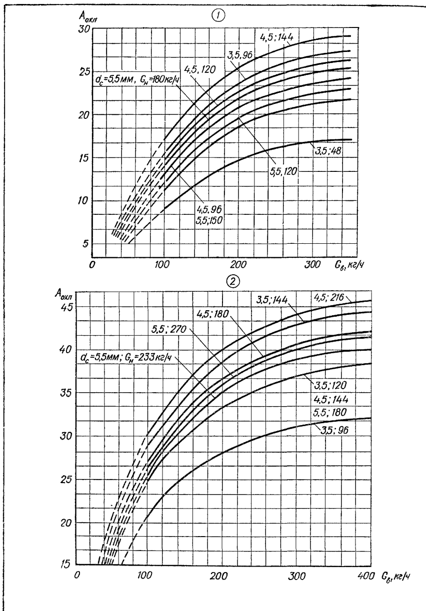
Лист VIII. 13. Удельный показатель A_{\text{охл}} в двухрядном теплообменнике ЭКД: 1 — типа КНЭ-У-0,8А; 2 — типа КНЭ-У-1,2.
