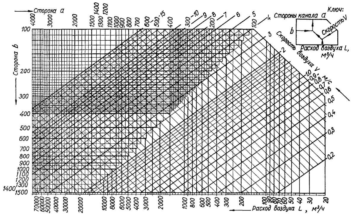
Лист VII.6. Номограмма для определения расходов воздуха и размеров прямоугольных каналов.
