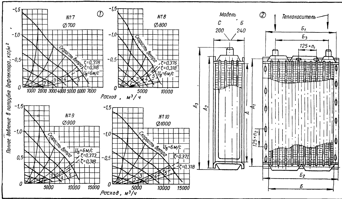
Лист VII.18. Аэродинамические характеристики дефлекторов УкрНИИСТ ДВК-5 № 7—10 (рис. 1) и многоходовых калориферов типа КВС, КВБ, КМС и КМБ (рис. 2).
